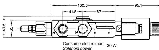
DETALLE CUERPO CON VÁLVULA PUESTA EN VACIO ELECTRICA DETAIL OF INLET COVER WITH UNLOADING VALVE
